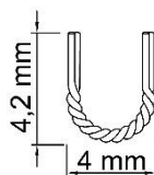
Dimensjoner: Klemmarkør
